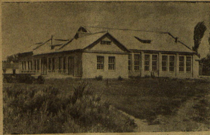
ВОЛЫНСКАЯ ОБЛАСТЬ. Построено новое здание для Торчинских машинно-тракторных мастерских. Заканчивается монтаж внутреннего оборудования. Основные цехи будут сданы в эксплуатацию к 32-й годовщине Великого Октября. На снимке: общий вид здания МТМ.
